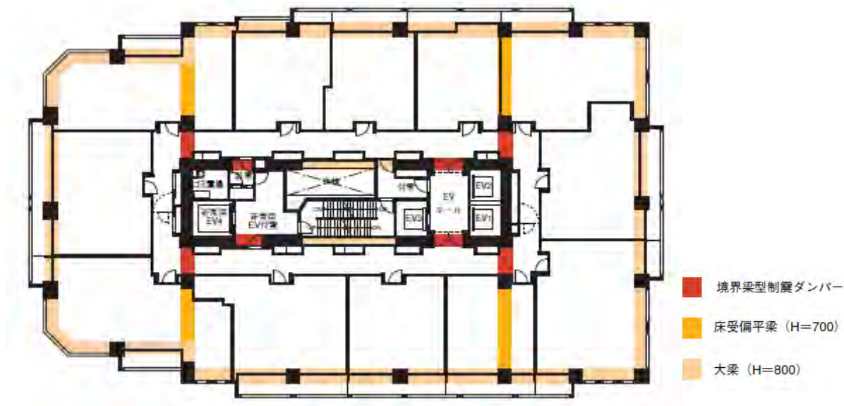
基準階架構計画図
