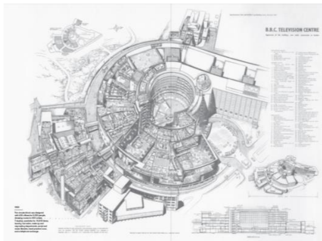
BBC放送局設計図(1958年当時)
