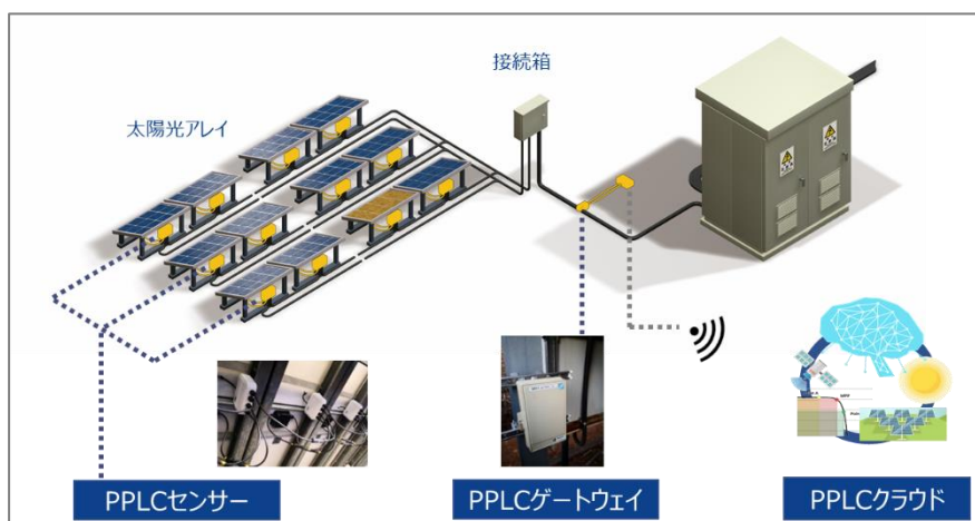
<太陽光発電設備の保守管理IoTプラットフォーム全体図>
