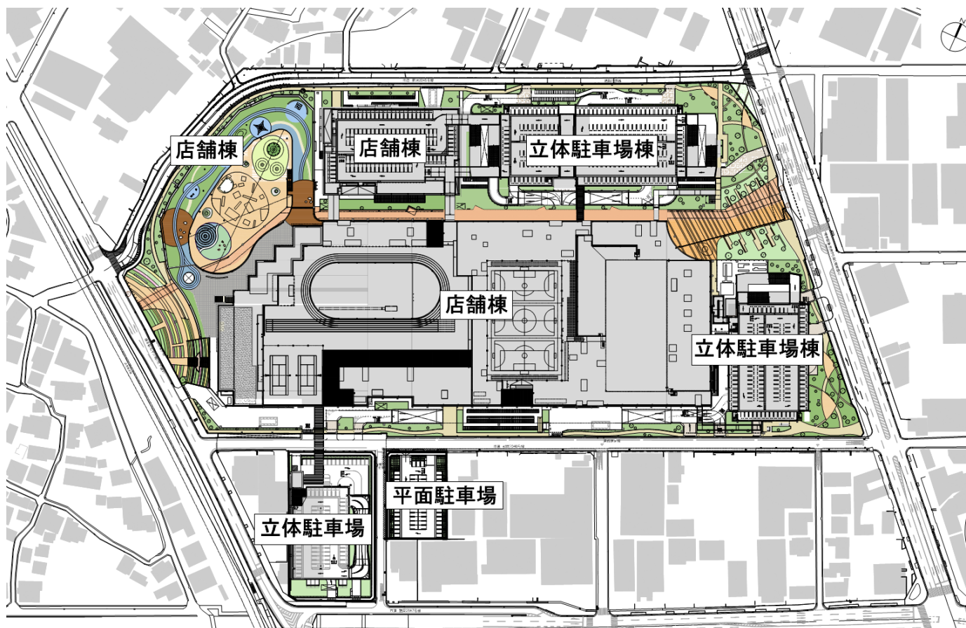
【建物配置図】
