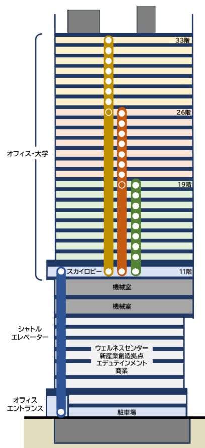
タワー棟断面
