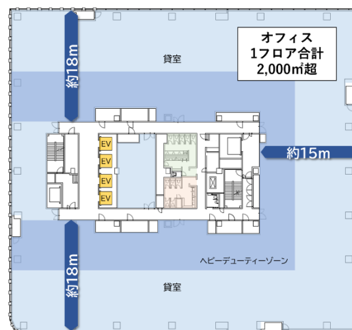
オフィス高層バンク平面
