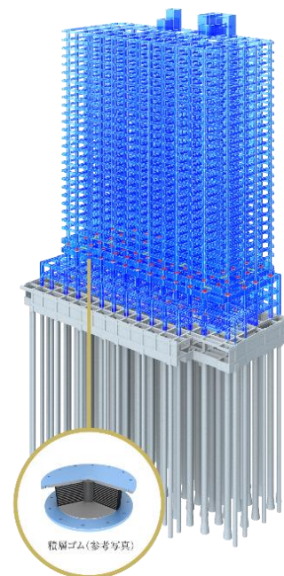
免震構造概念図
