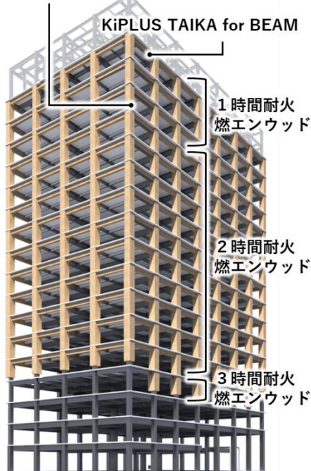
構造概要
